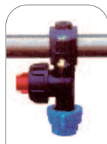
Jet avec ecrou accouplement rapide et antigoutte a membrane
